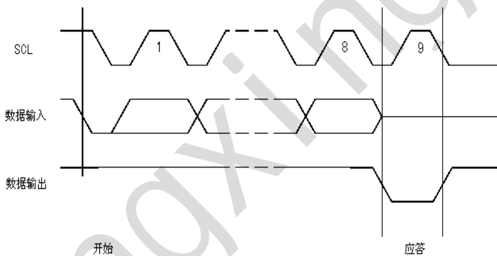
图 7、输出响应
