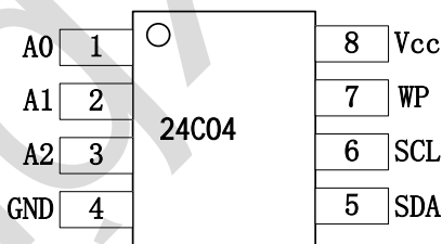
图 2、引脚排列图
