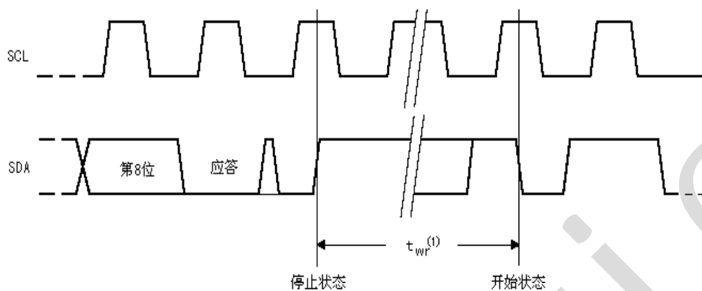
图 6、写周期时序
