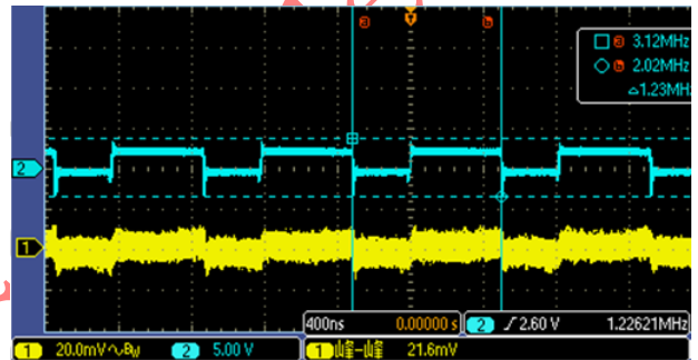
VIN = 2.7V, ILOAD = 1A Waveform
