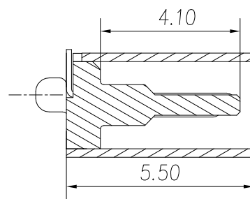
剖面: A-A
