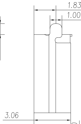
剖面: A-A
