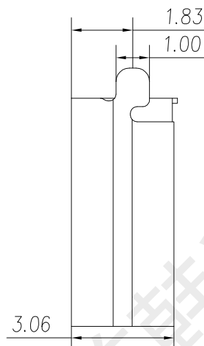
剖面: A-A
