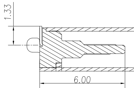
剖面: A-A
