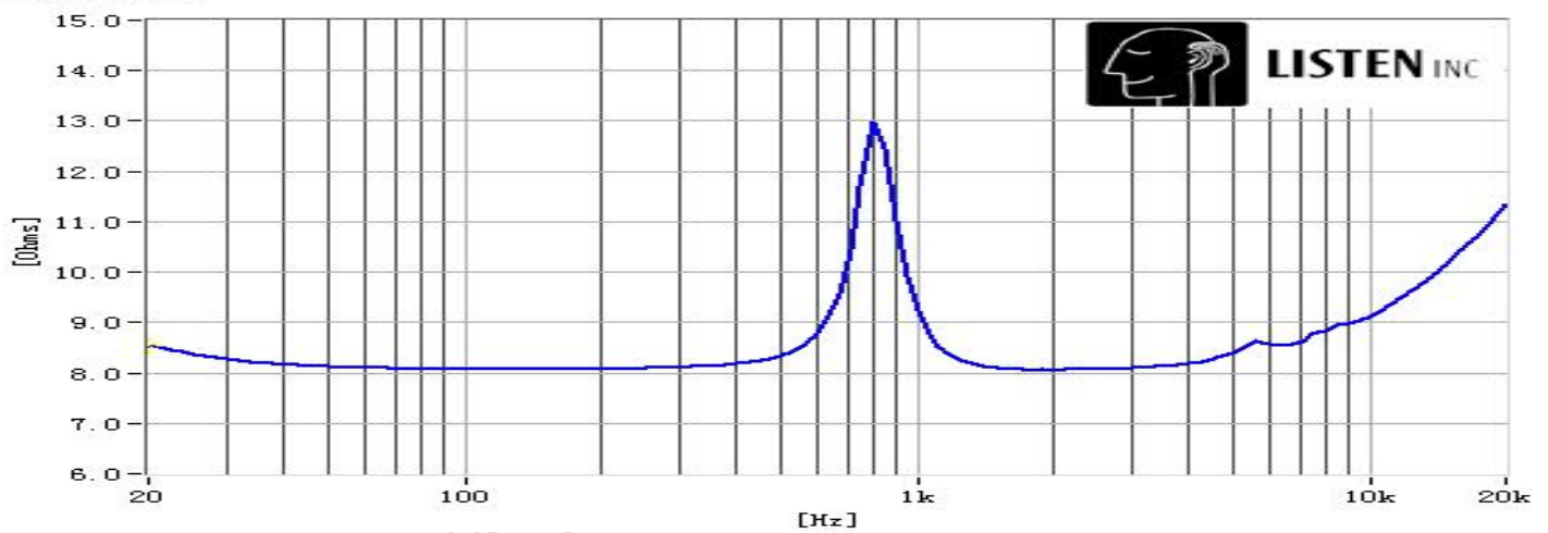
阻抗曲线
