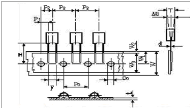
Fig.1 P=5.0/7.5mm
