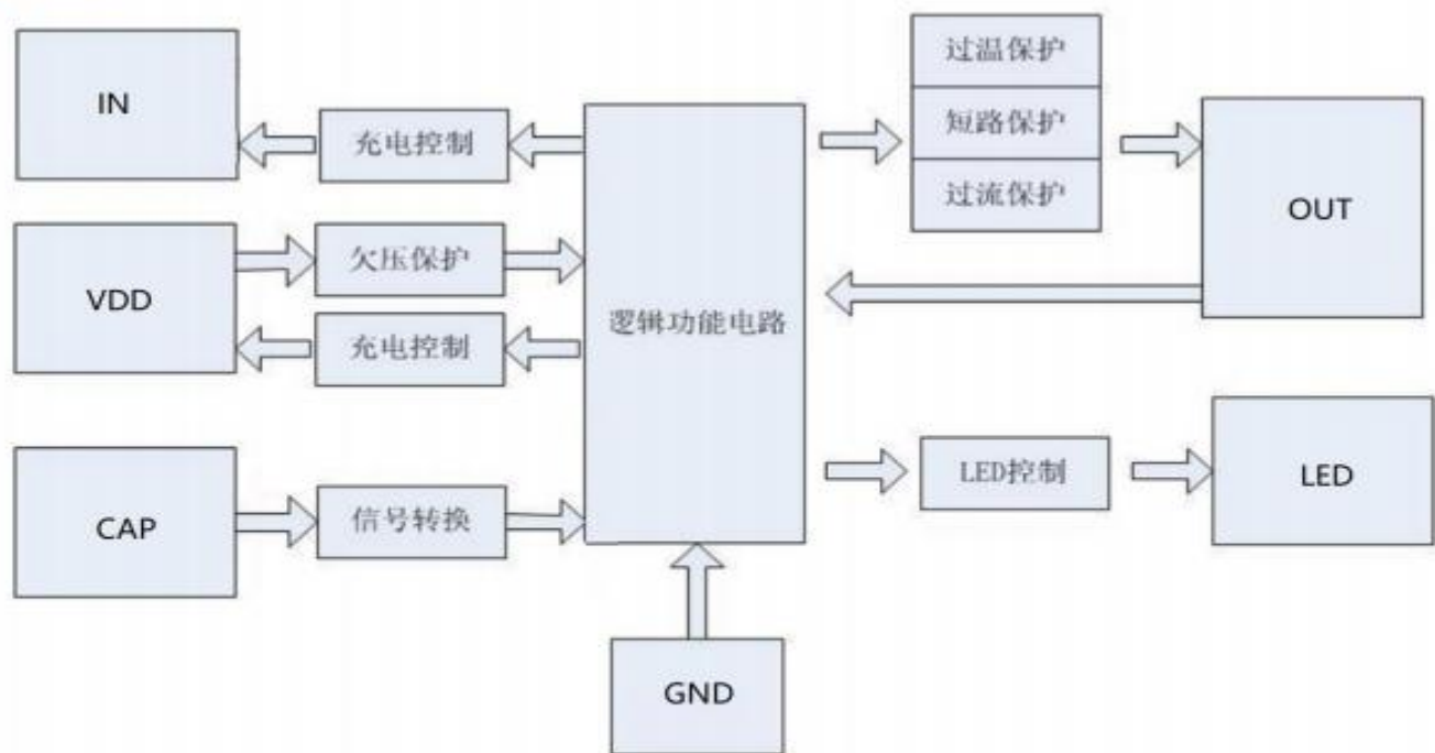
功能方框图
