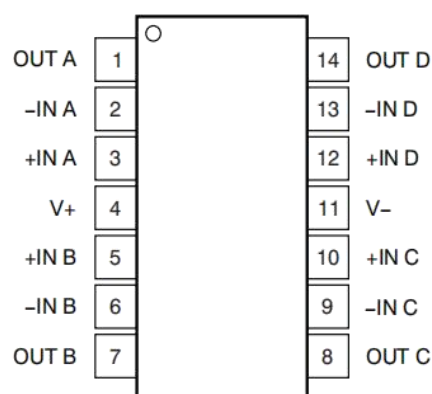
TLV4333A TSSOP-14(俯视图)
