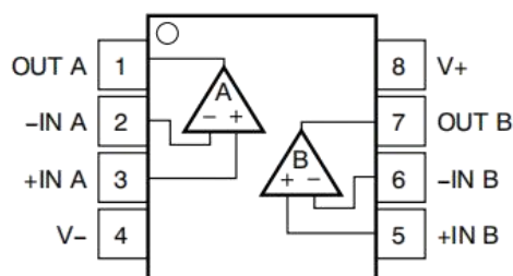
TLV2333A SOP-8/MSOP-8 俯视图
