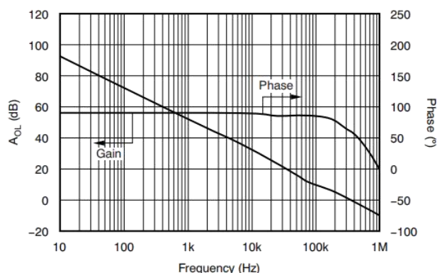
Figure 2. 开环增益与频率间的关系
