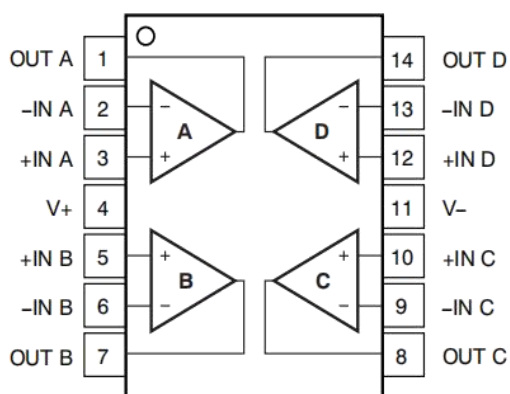
TLV4333A SOP-14(俯视图)
