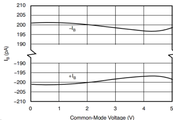
Figure 6. 输入偏置电流与共模电压间的关系
