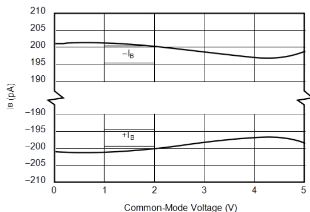
Figure 6. 输入偏置电流与共模电压间的关系
