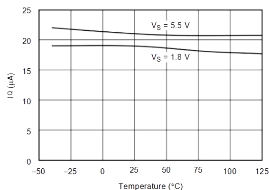
Figure 8. 静态电流与温度间的关系
