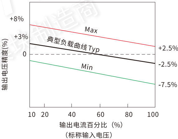
误差包络曲线图 其它输出
