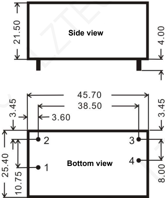
单位 Unit: mm 公差 Tolerance: \pm 0.5\text{mm}
