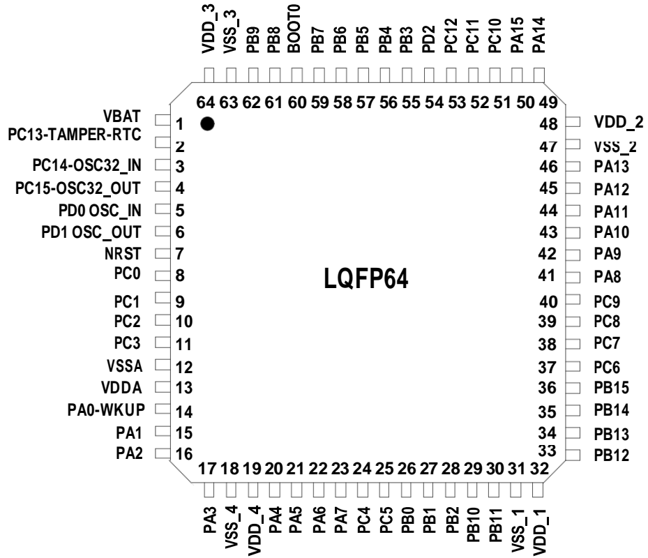
引脚分布图
