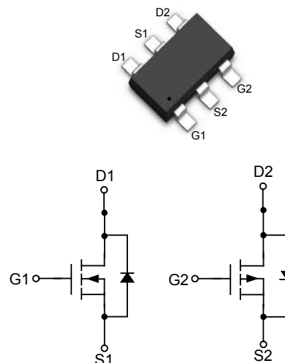
N+P MOSFET
