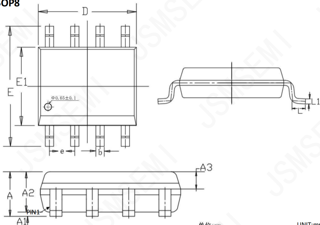
SOP8
