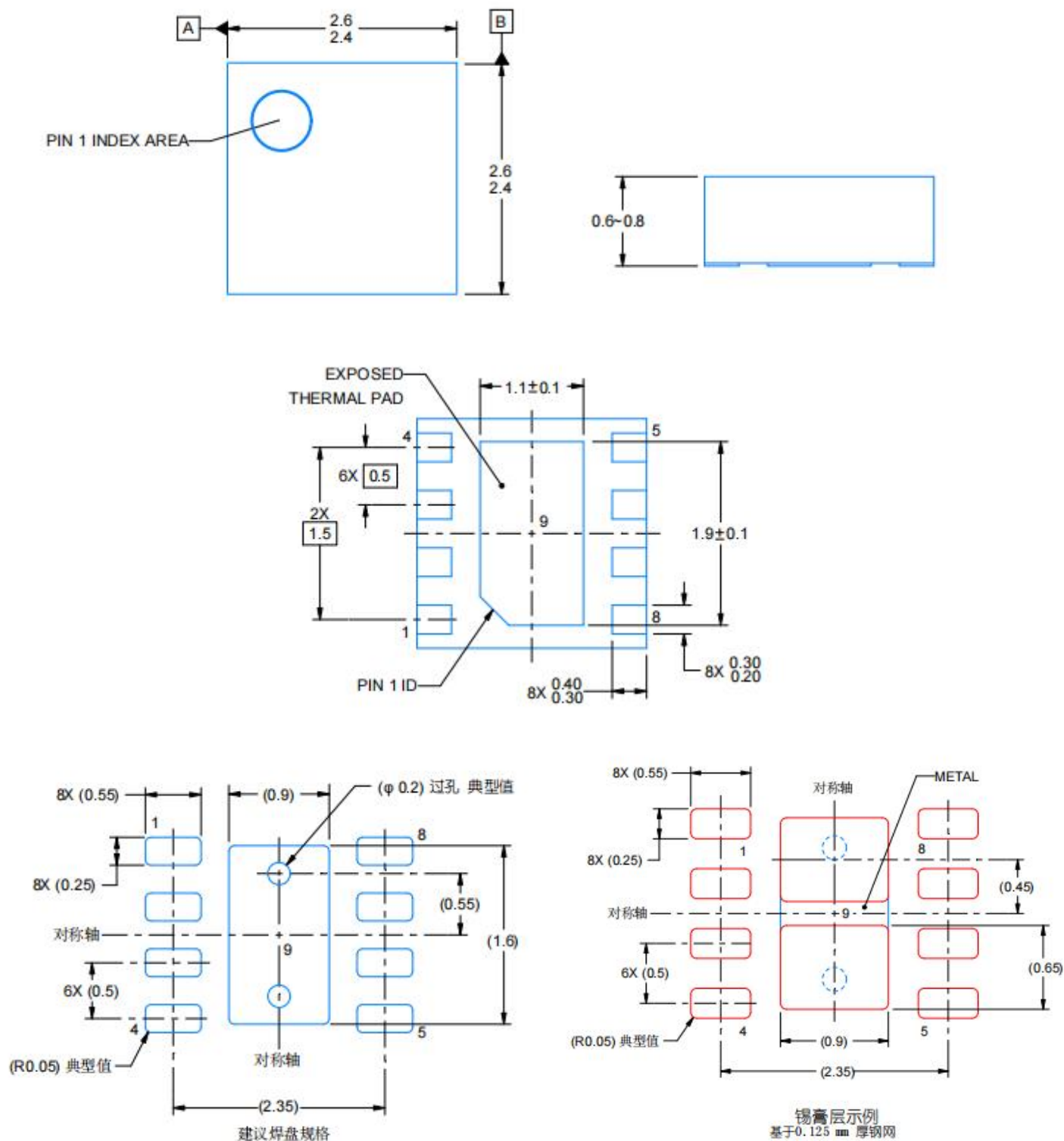
图 13.2 PCB 焊盘引脚尺寸图
