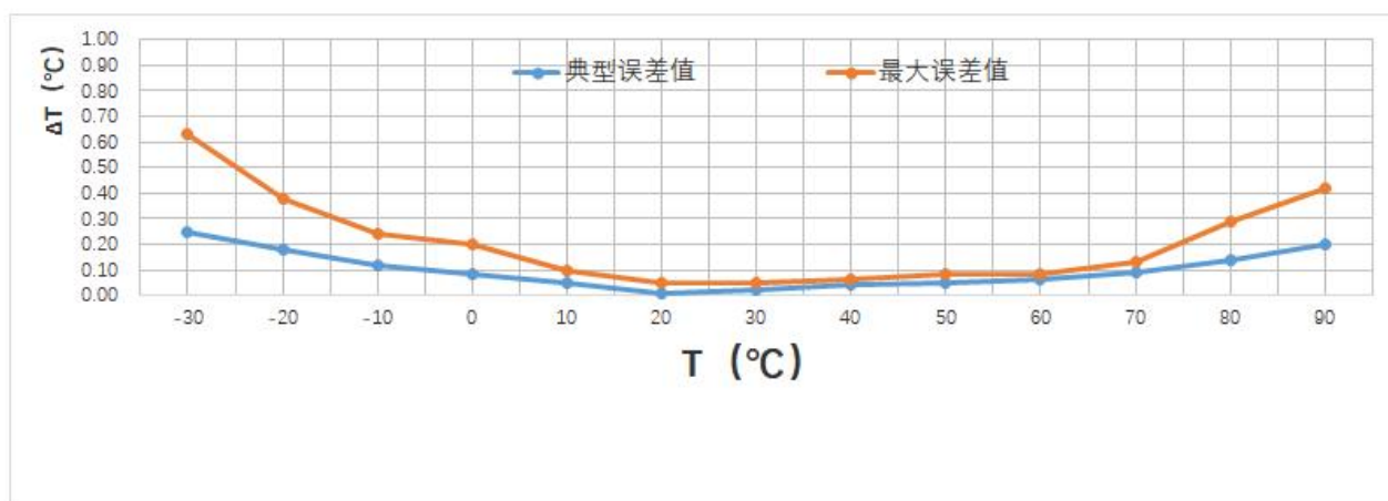
图 7- 3 MTS01W 精度误差曲线
