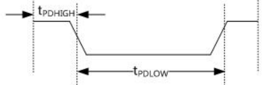
图 11.10 时隙图
