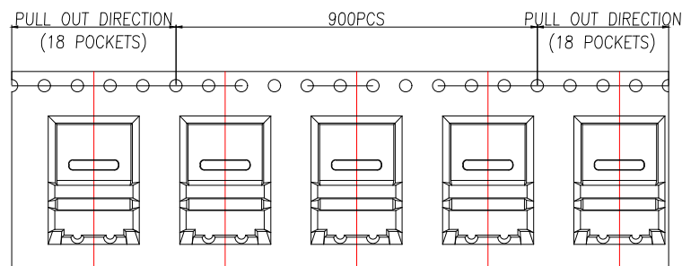
① 产品入载带示意图
