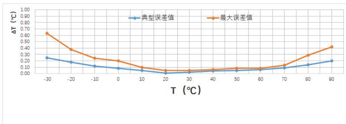
图 7-3 M117W 精度误差曲线
