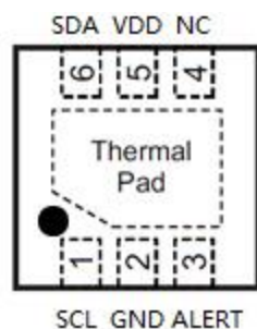
(正面透视图)
