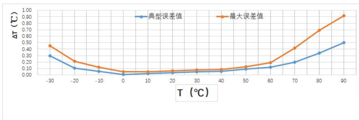
图 7-2 M117Z 精度误差曲线
