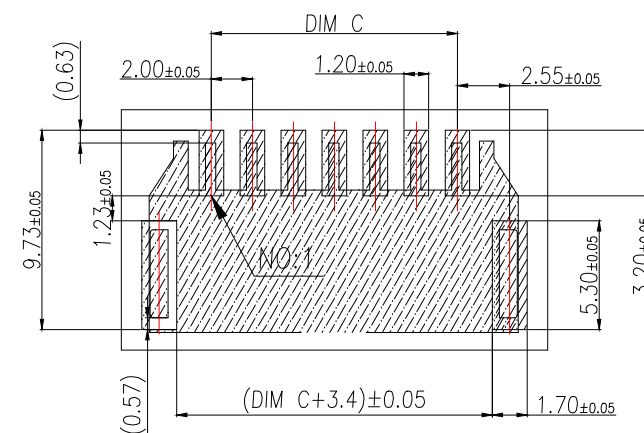
适用线路板(PCB LAYOUT)
