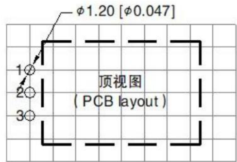
PCB 印刷版图
