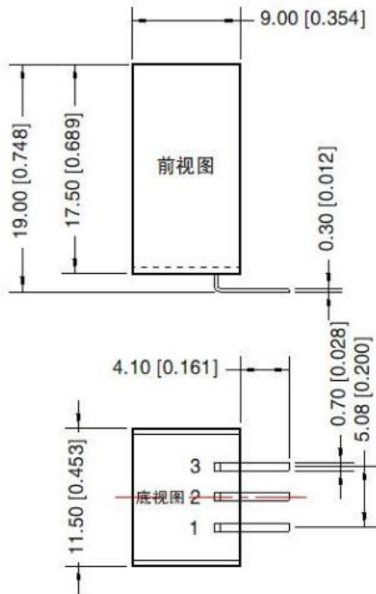
外观尺寸图
