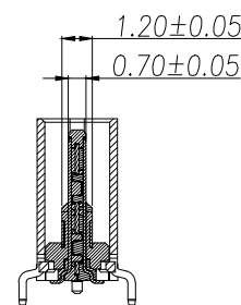
SECTION A-A
