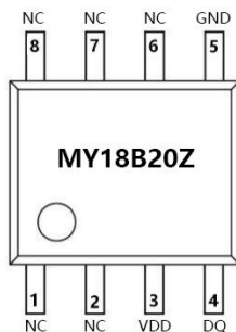
正视图
