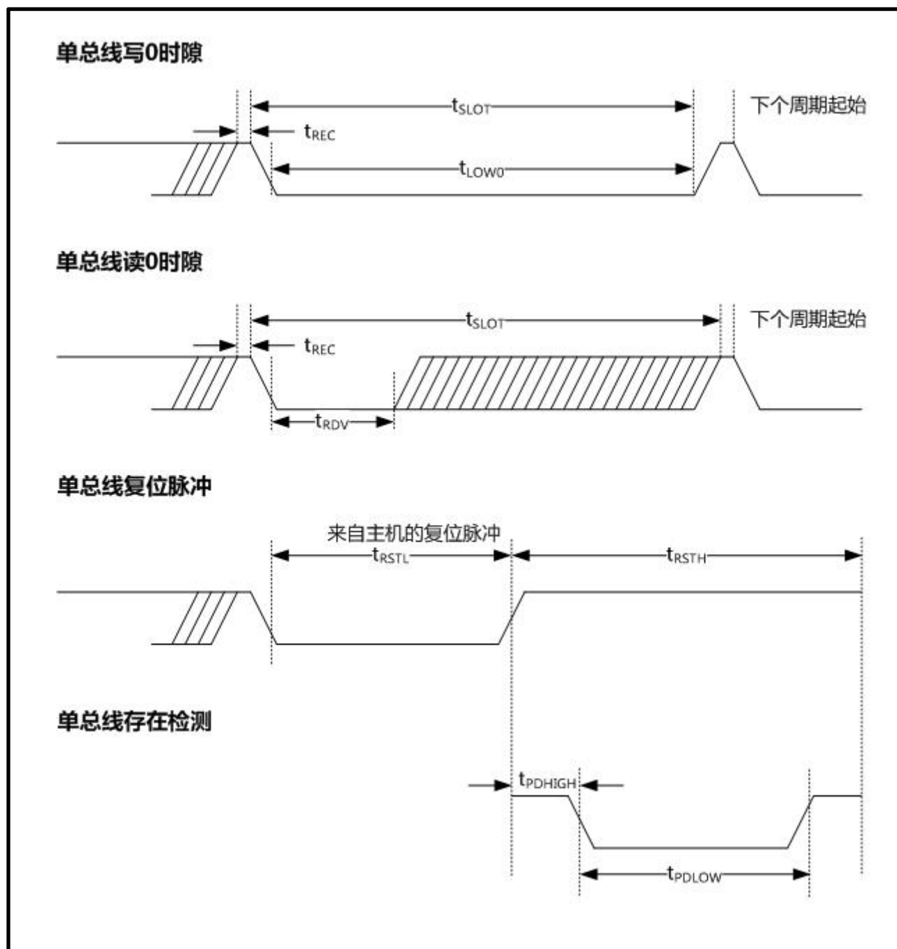
图 10.6-5 时序图
