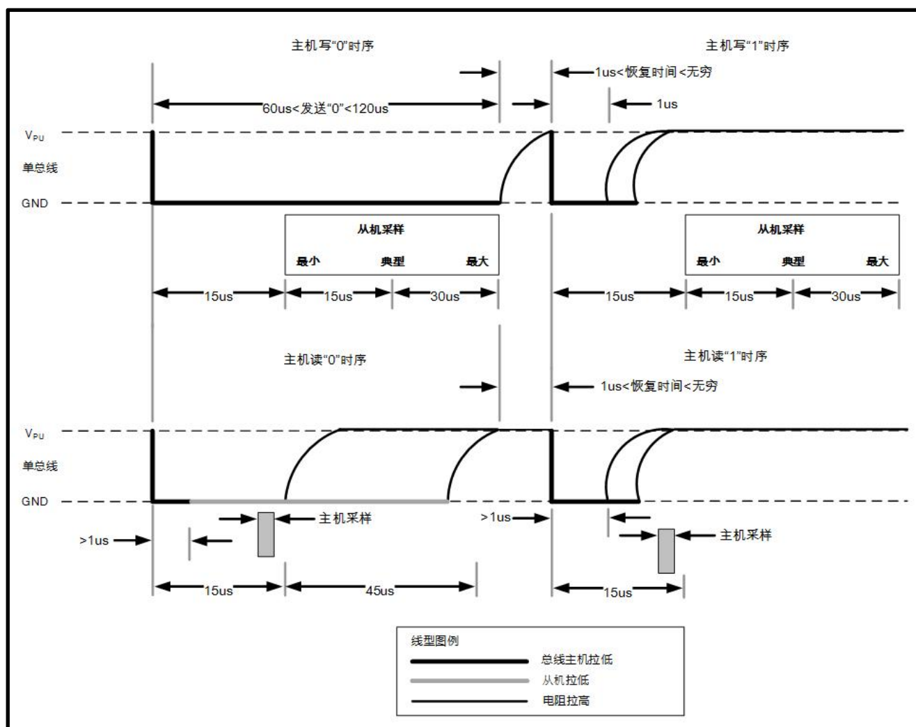
图 10.6-2 读/写时序
