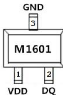
正视图
