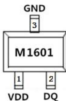
正视图
