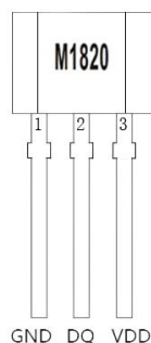
正视图
