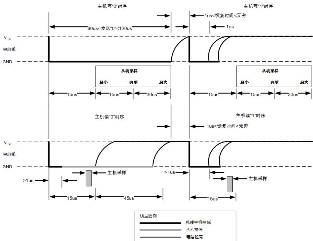
图 11.7-2 读/写时序
