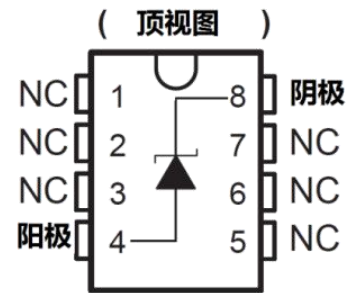
图 4 SOP8/MSOP8 管脚图
