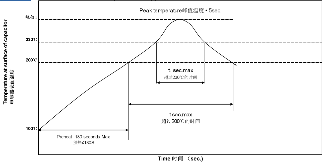
For Liquid SMD Type 回流焊温度曲线图-贴片固态电容器
