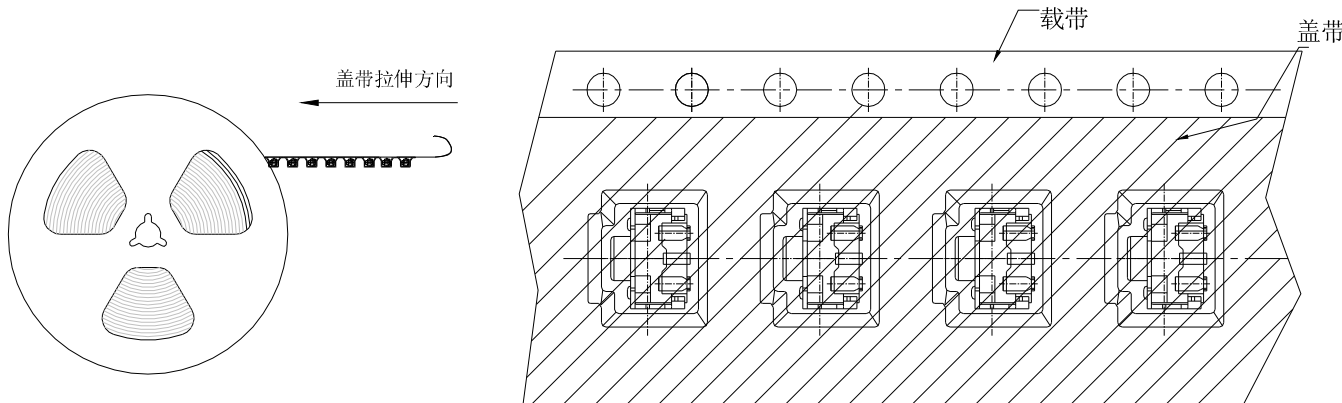
包装图
