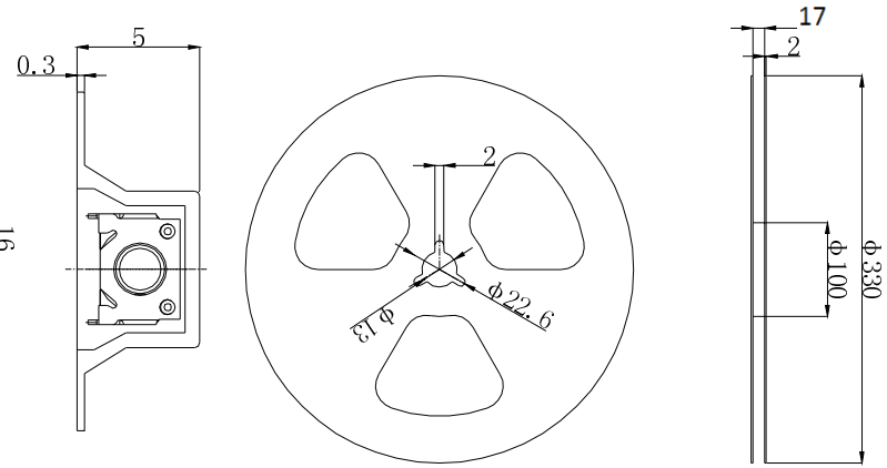
编带盘尺寸图
