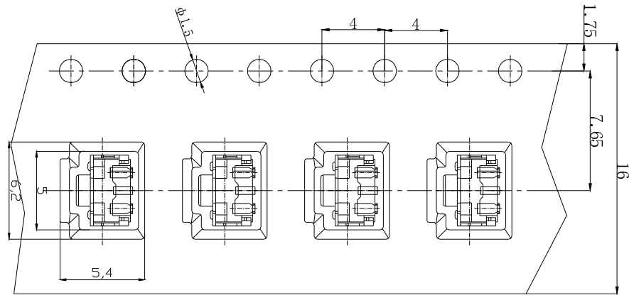
载带尺寸图
