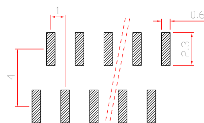
安装尺寸
