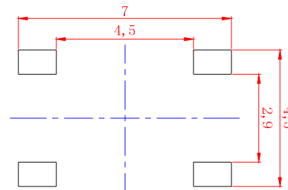
P C B 参考图
