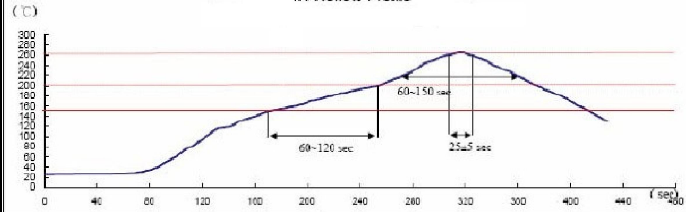
IR-Reflow Profile
