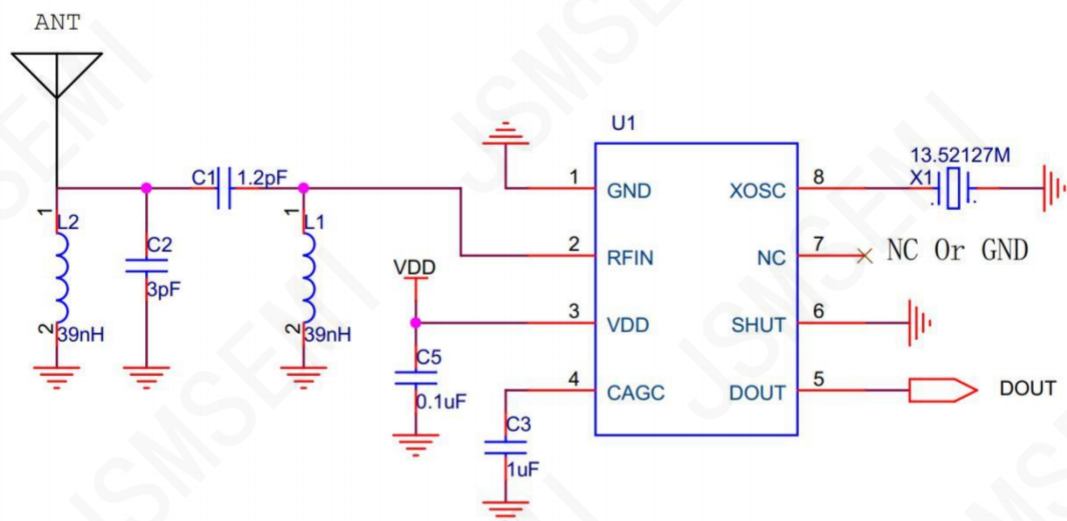
JSM903R-433M典型应用原理图
