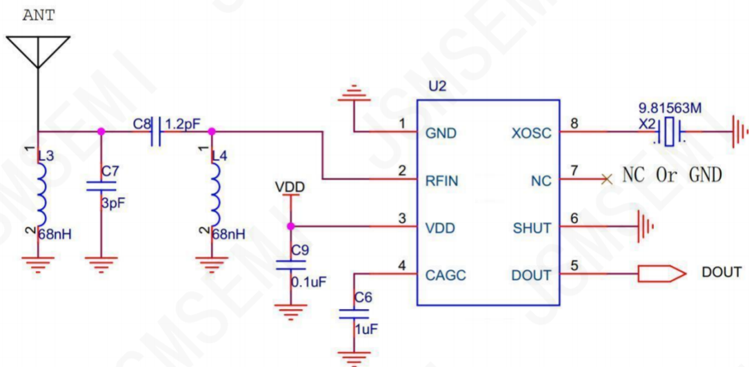
JSM903R-315M典型应用原理图
