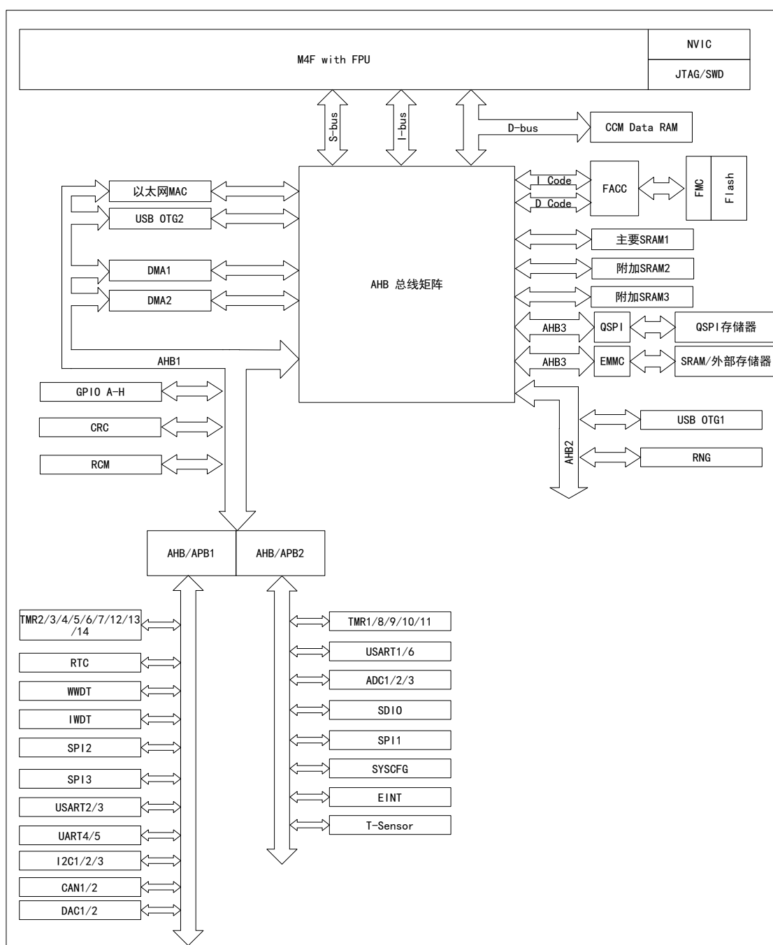
图 7 APM32F427xG_F425xG_F423xG 系统框图
