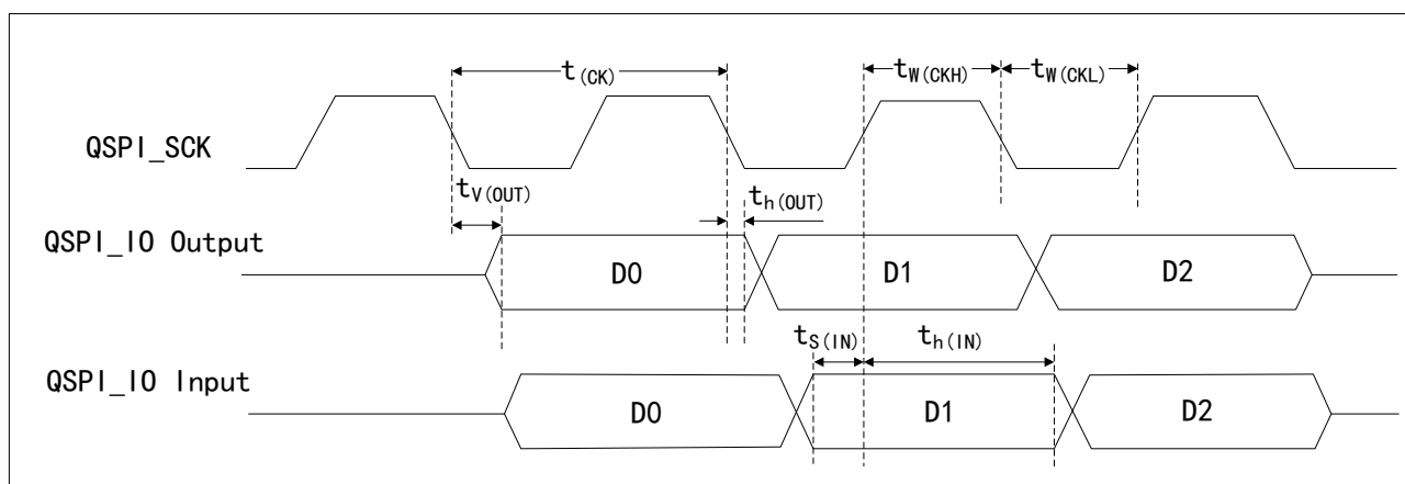
图 18 QSPI 时序图
