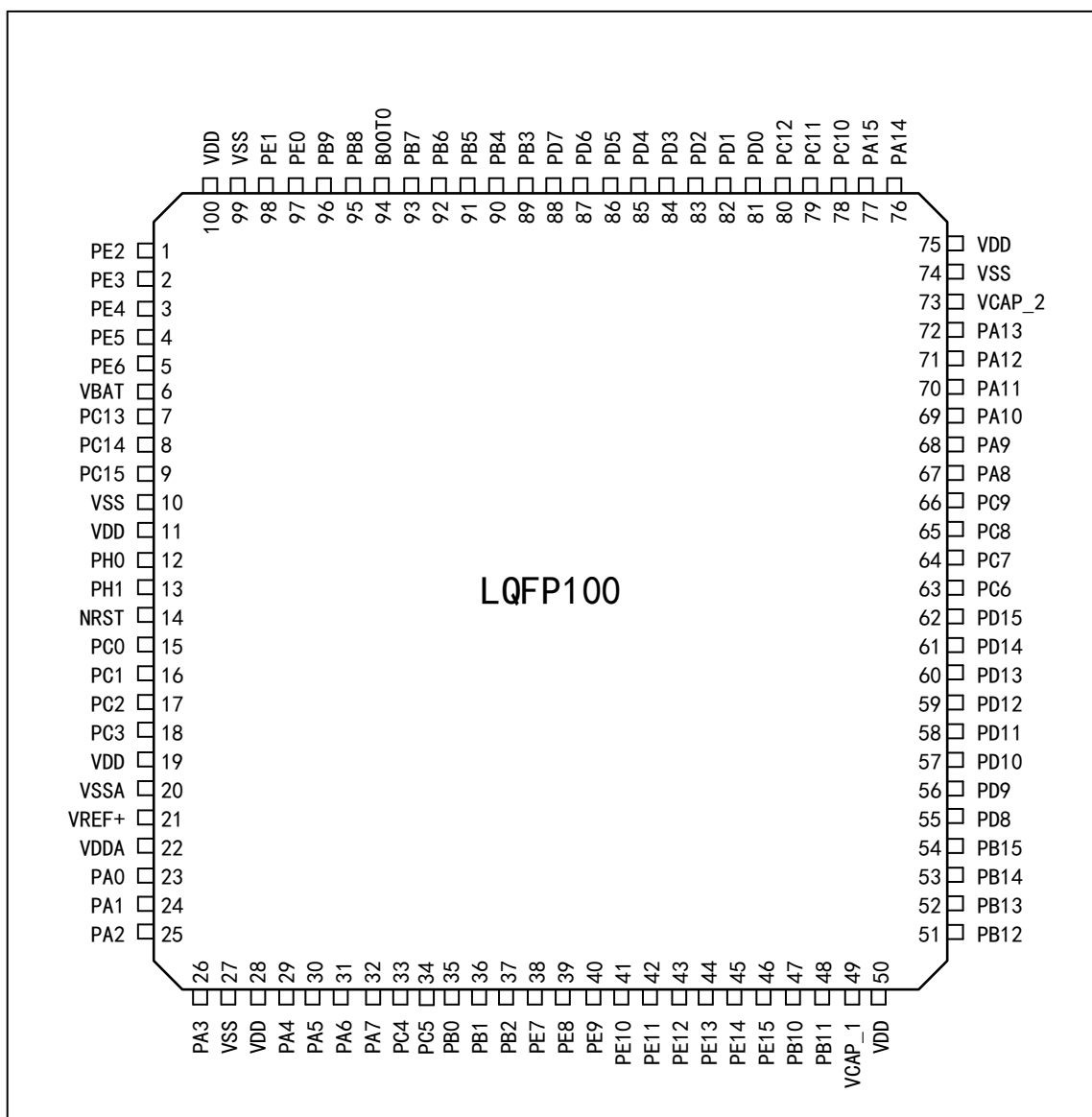
图 2 APM32F427xG_F425xG_F423xG 系列 LQFP100 引脚分布图
