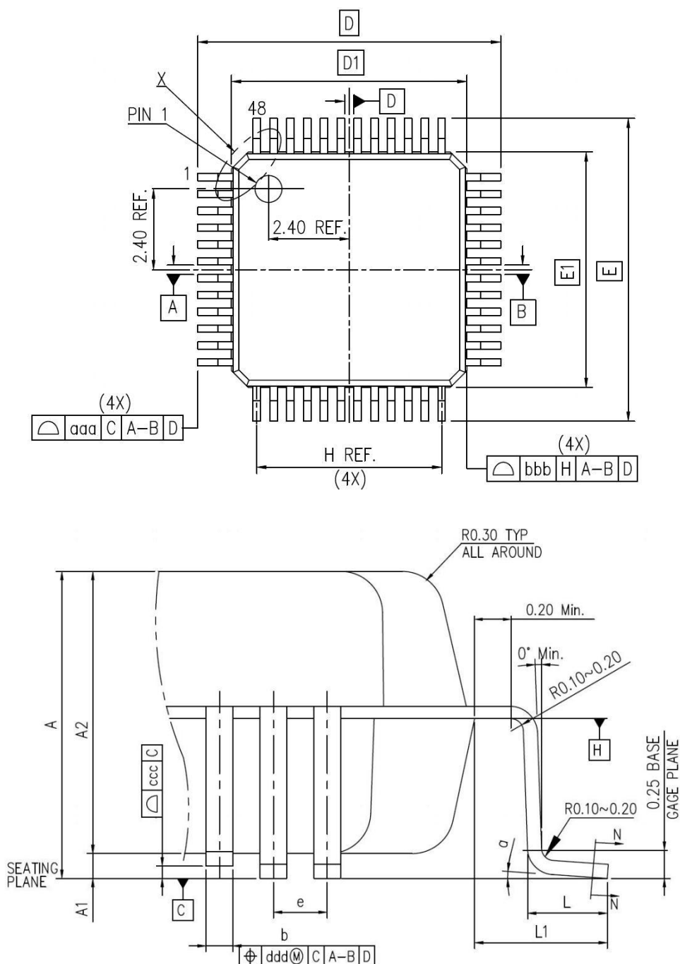
图 25 LQFP48 封装图
