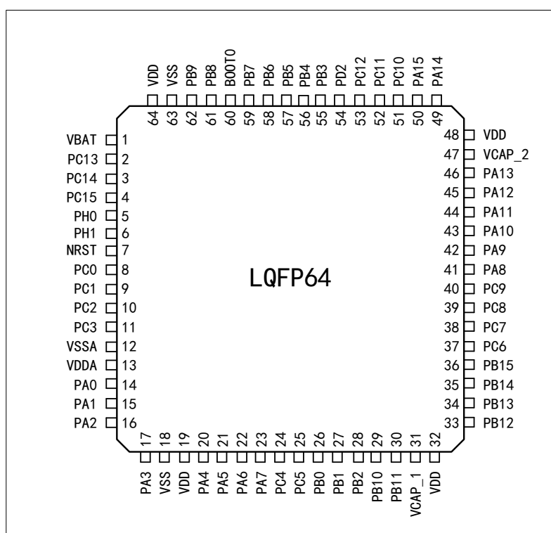
图 3 APM32F427xG_F425xG_F423xG 系列 LQFP64 引脚分布图
