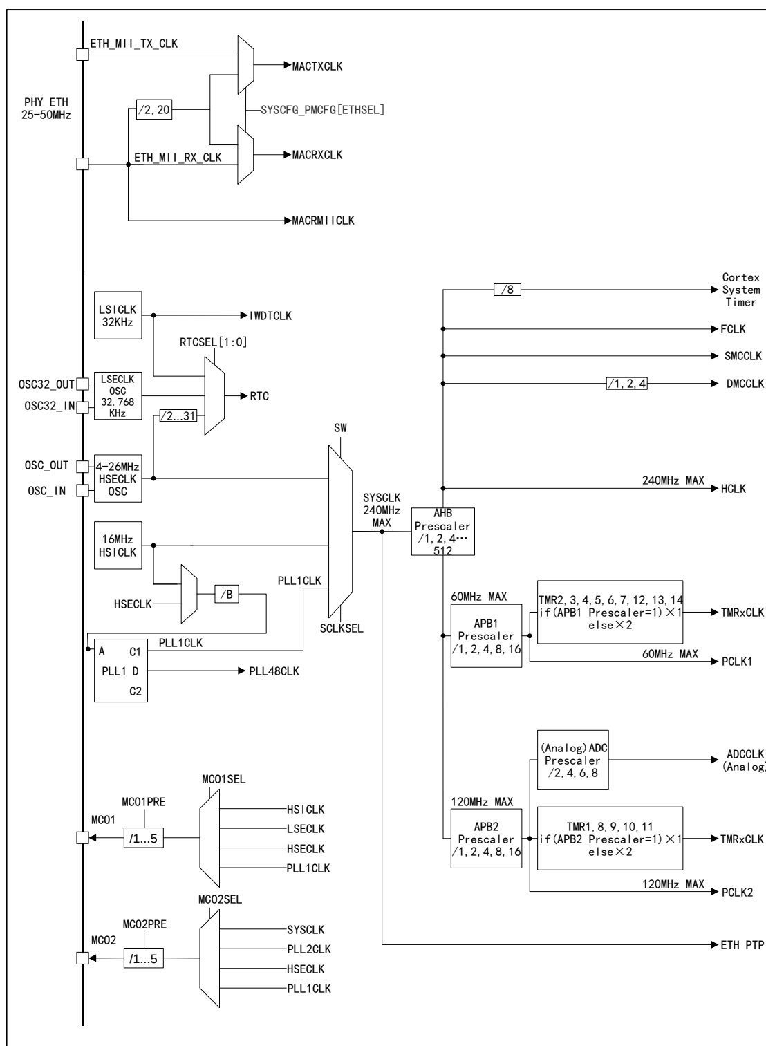
图 8 APM32F427xG_F425xG_F423xG 时钟树
