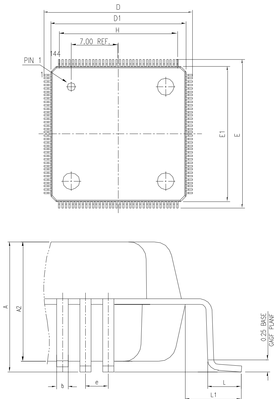
图 19 LQFP144 封装图
