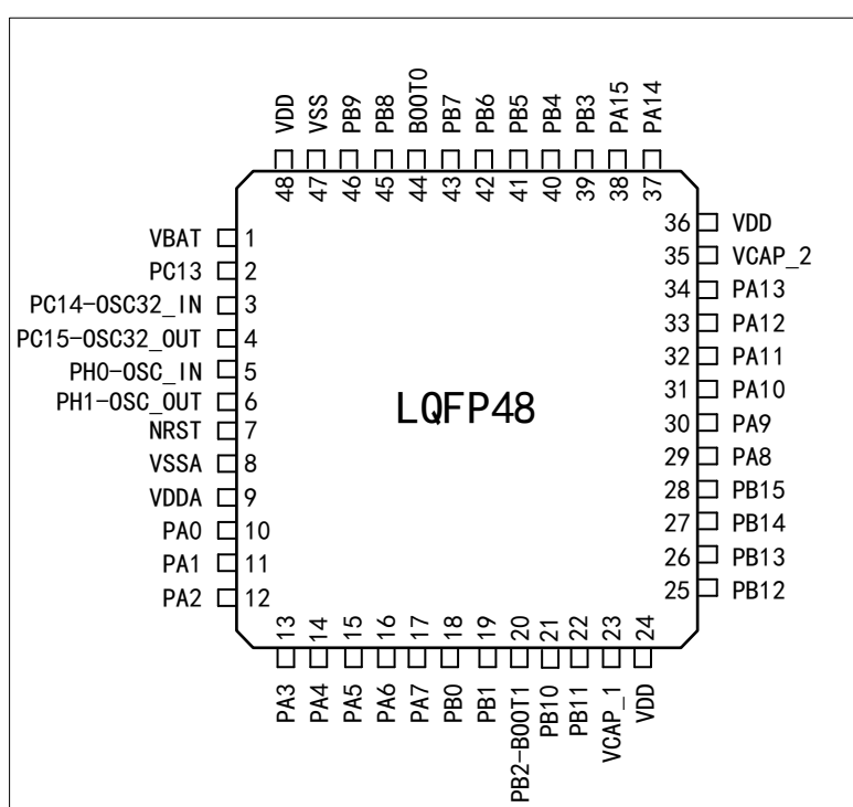
图 4 APM32F427xG_F425xG_F423xG 系列 LQFP48 引脚分布图
