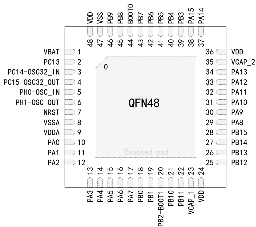
图 6 APM32F427xG_F425xG_F423xG 系列 QFN48 引脚分布图
