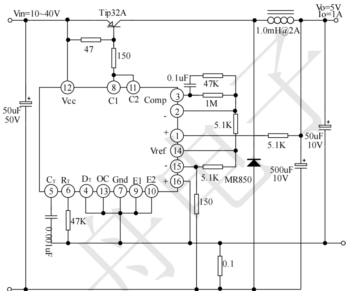
图 12 脉宽调制降压式转换器
