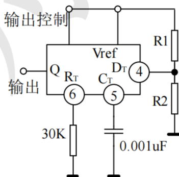
图 9 死区时间控制电路
