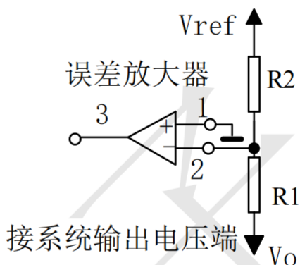
图 6 误差放大器传感技术 负输出电压: V_o = V_{ref} * R_1/R_2
