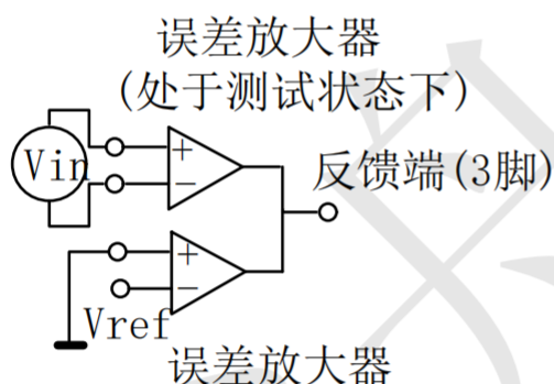
图 1 误差放大器特性
