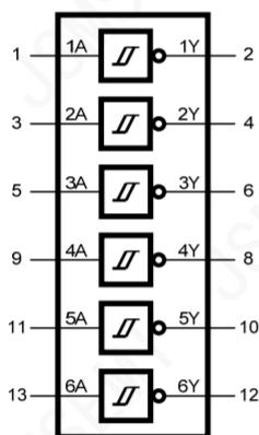
图 1 逻辑符号
