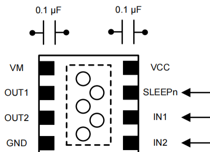
图 8-2 PCB 示意图
