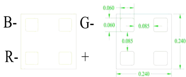
焊盘面图示
