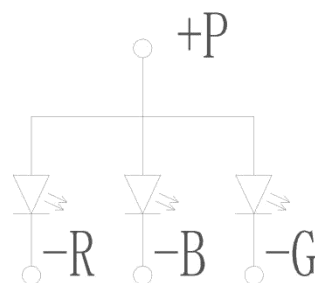
电路图
