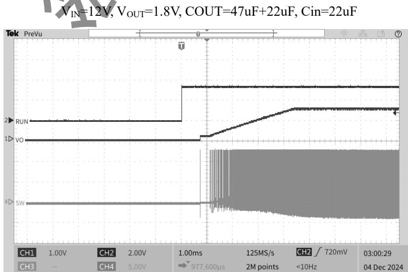
图 11 空载启动
