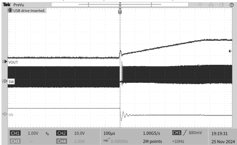
图 15 短路恢复
