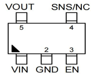
TSOT-23-5
