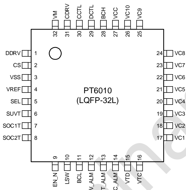
图 5. 管脚定义图
