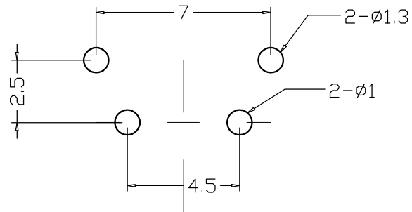
PCB线路版图
