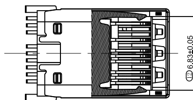
剖面: B-B
