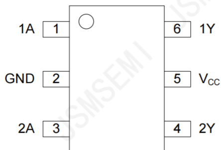
SOT23-6/SOT363
