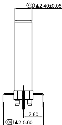
截面 A-A
