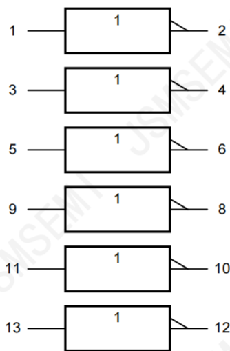
图 2 IEC 逻辑符号
