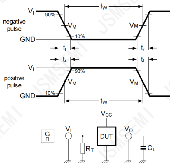
图4 测量开关时间的测试电路
