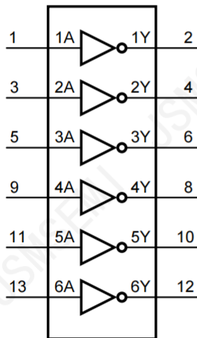
图 1 逻辑符号
