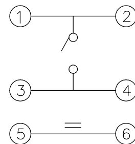
电路图
