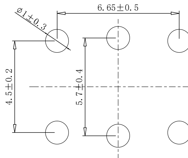
推荐PCB线路板图
