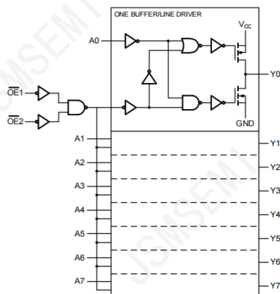
图 4 逻辑框图
