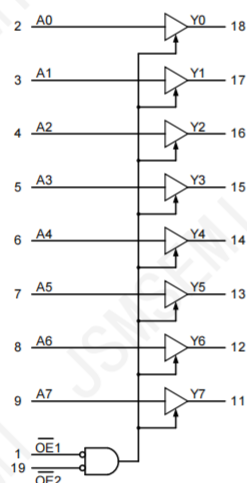
图 1 逻辑符号
