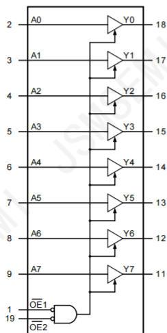
图 3 功能框图
