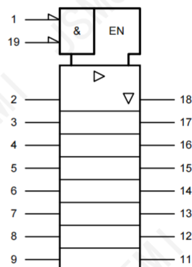
图 2 IEC 逻辑符号
