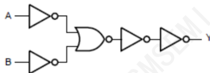
图 3 逻辑框图
