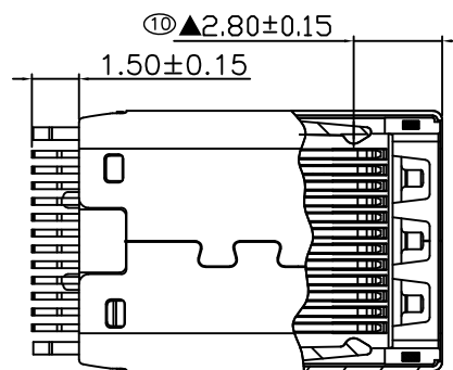
截面 B-B
