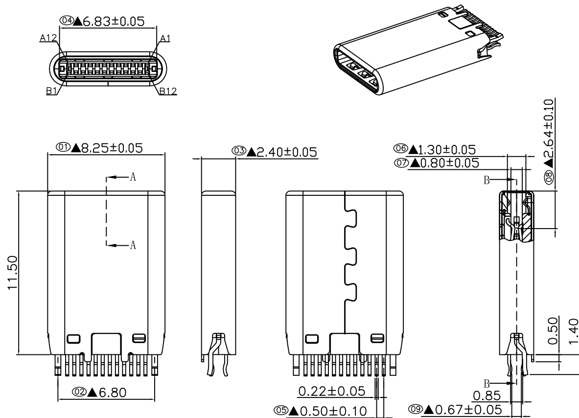
截面 A-A
