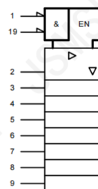
图 2 IEC 逻辑符号
