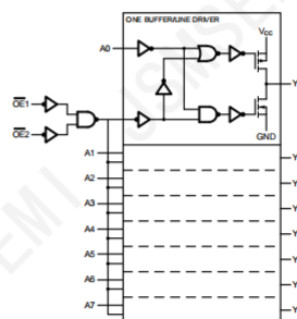
图 4 逻辑框图
