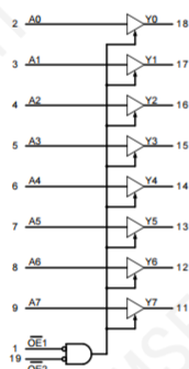
图 1 逻辑符号
