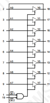
图 3 功能框图
