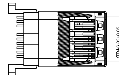
剖面: B-B
